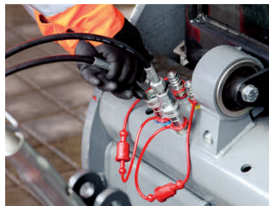
TransGiant är utrustad med lättåtkomliga hydraulanslutningar vid redskapsbyte.
